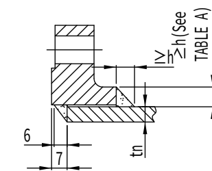
法兰与接管焊接视图
