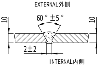
纵环焊缝焊接视图
