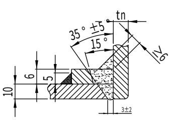
有补强圈接管焊接视图 N1、N5
