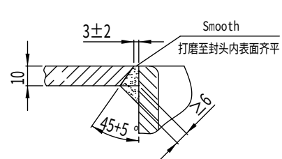
接管N6焊接视图
