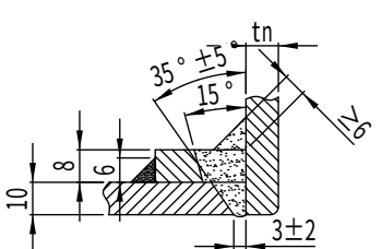
有补强圈接管焊接视图 N4
