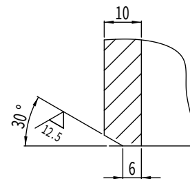
Detail I (详图 I)
